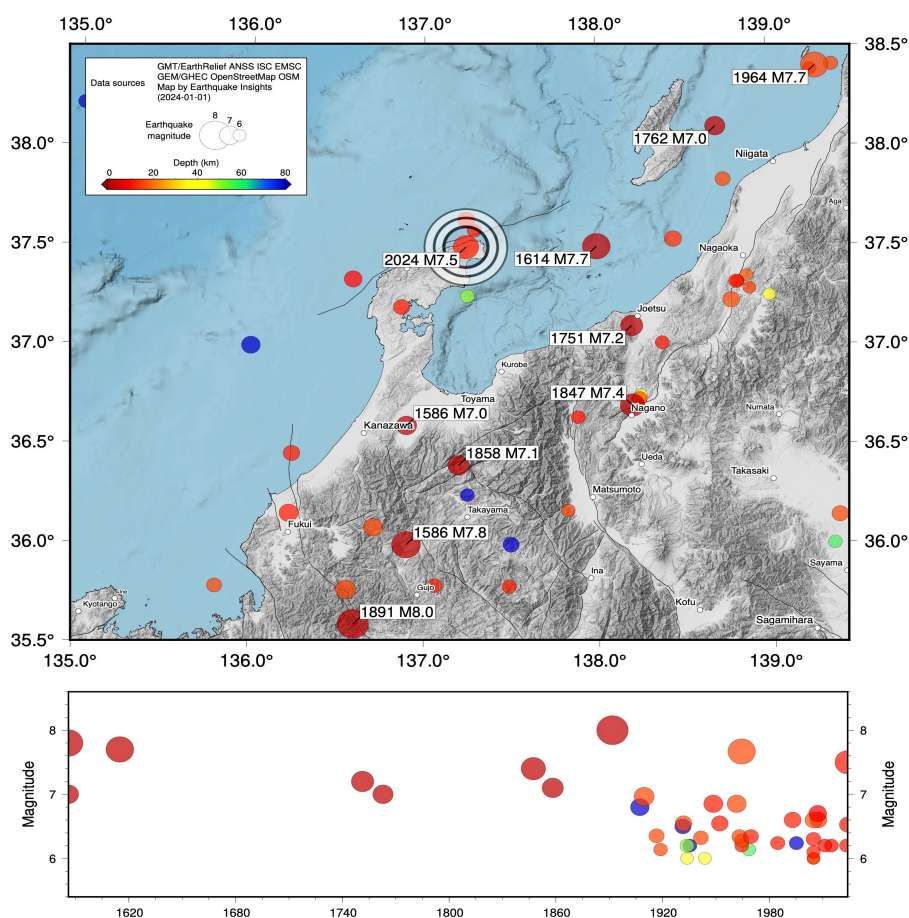
شکل ۱- زمین لرزه های رخ داده تاریخی در ژاپن (برگرفته از GHEC)
