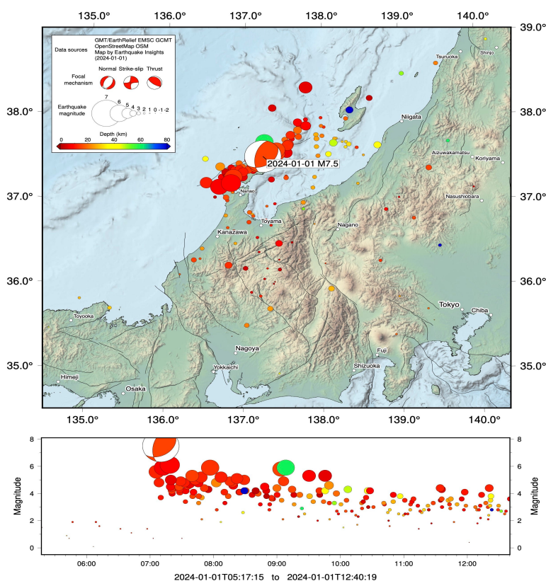
شکل ۳- ساز و کار کانونی زمین لرزه
